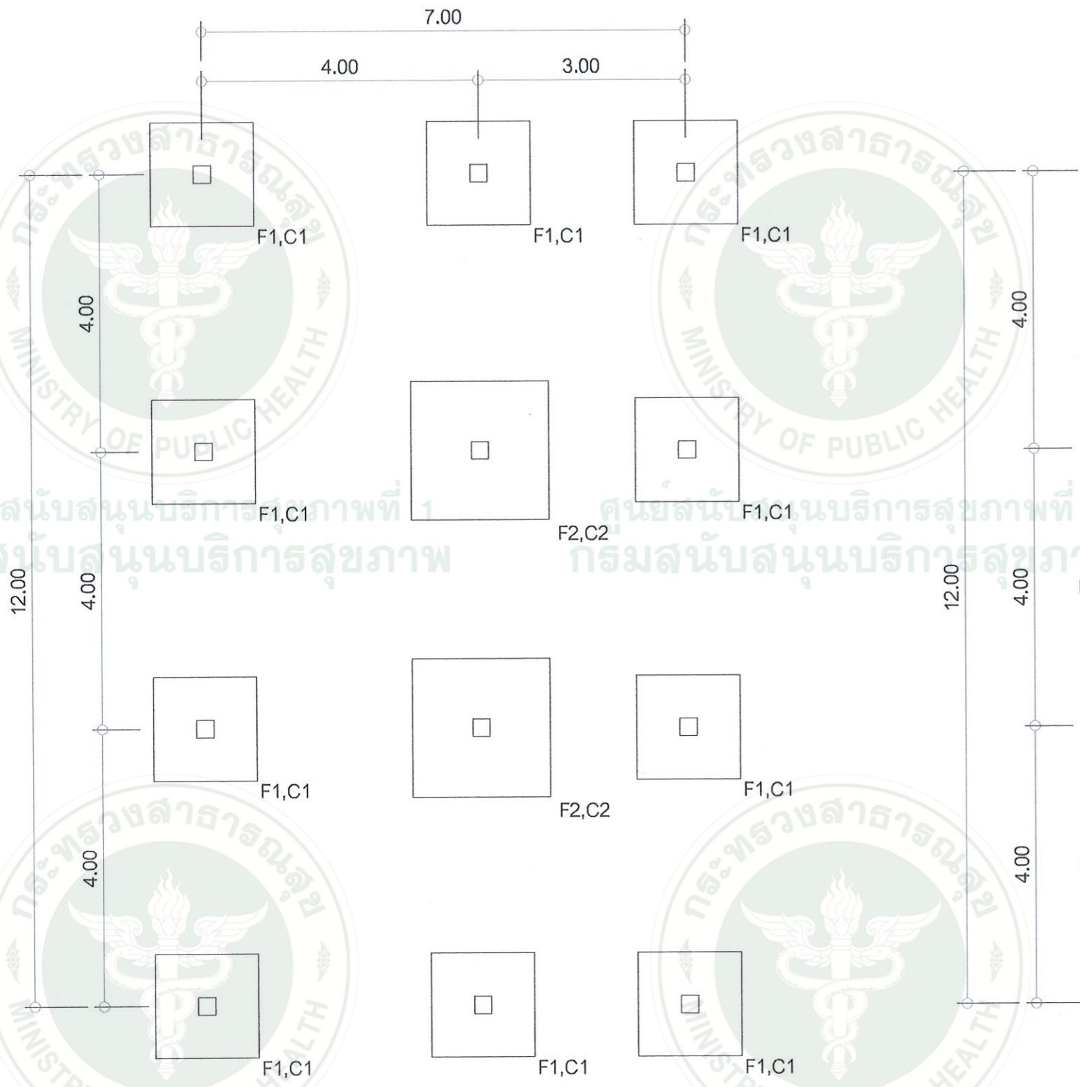
ผังโครงสร้างฐานราก
