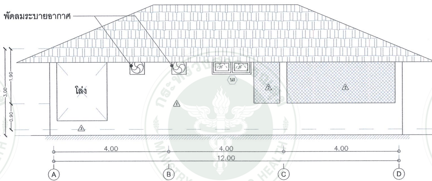
รูปด้าน 2
