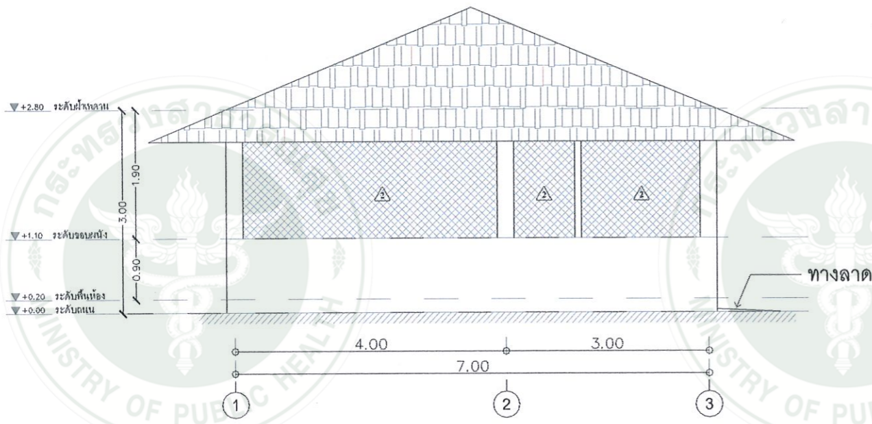
รูปด้าน 3
